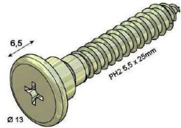
TORNILLO por TAPÓN para sujetar tapón y placa en el tubo
