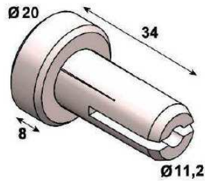
TAPÓN DE NYLON a expansión para tubo Ø 14mm
