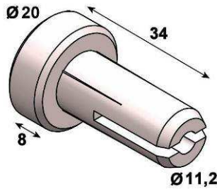
TAPPO IN NYLON ad espansione per tubo \varnothing 14 \times 1,2 \text{mm}
